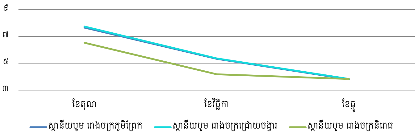
ក្រាហ្វិចខាងក្រោមឆ្លុះបញ្ចាំងពីកម្រិតទឹកទន្លេ ពីខែតុលា ដល់ខែធ្នូ ឆ្នាំ២០១៤ (គិតជាប្រវែងម៉ែត្រ)
